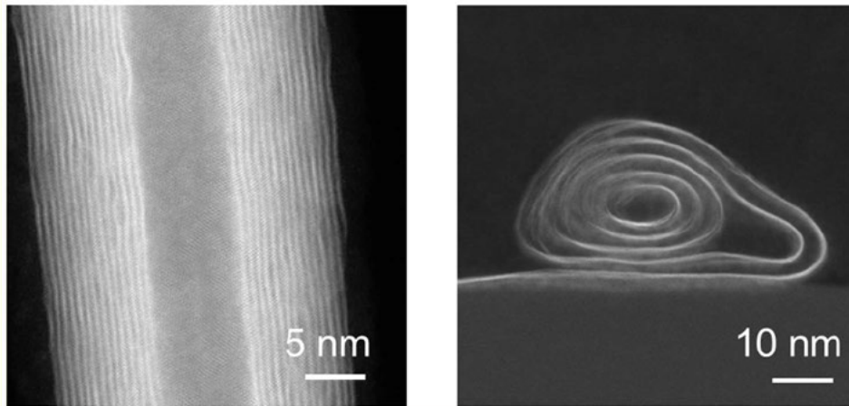
図2 ナノスクロールの電子顕微鏡写真。
