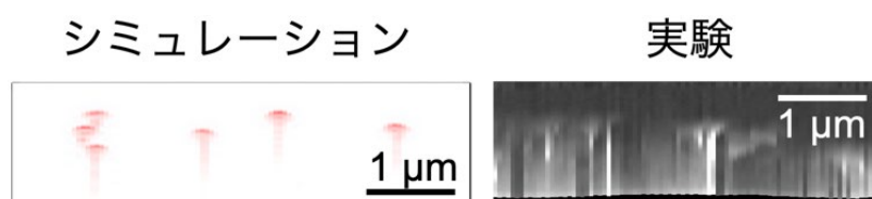
図3：生体高分子（アクチン繊維）のシミュレートされた3次元原子間力顕微鏡像（左）と実験により計測された像（右）。図1, 2で開発した計算手法で、単純な直線状構造と分かっているアクチン繊維の実験を再現できるかを確認している。実験では下に引き伸ばされた三角の形状が観測されており、この形状はシミュレーションでも再現されている。
