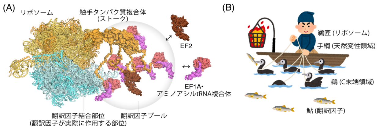
図 3. 本研究のまとめ図
