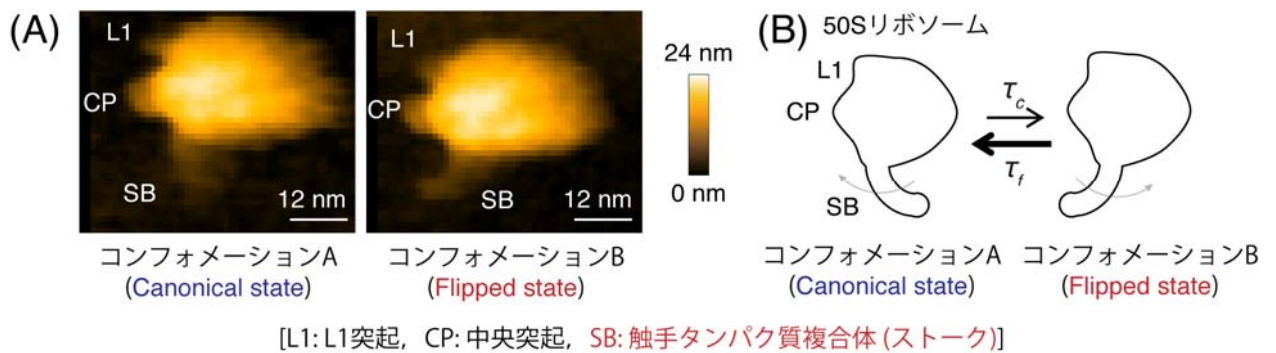
図 1. 高速 AFM によって可視化された触手タンパク質複合体の動態
