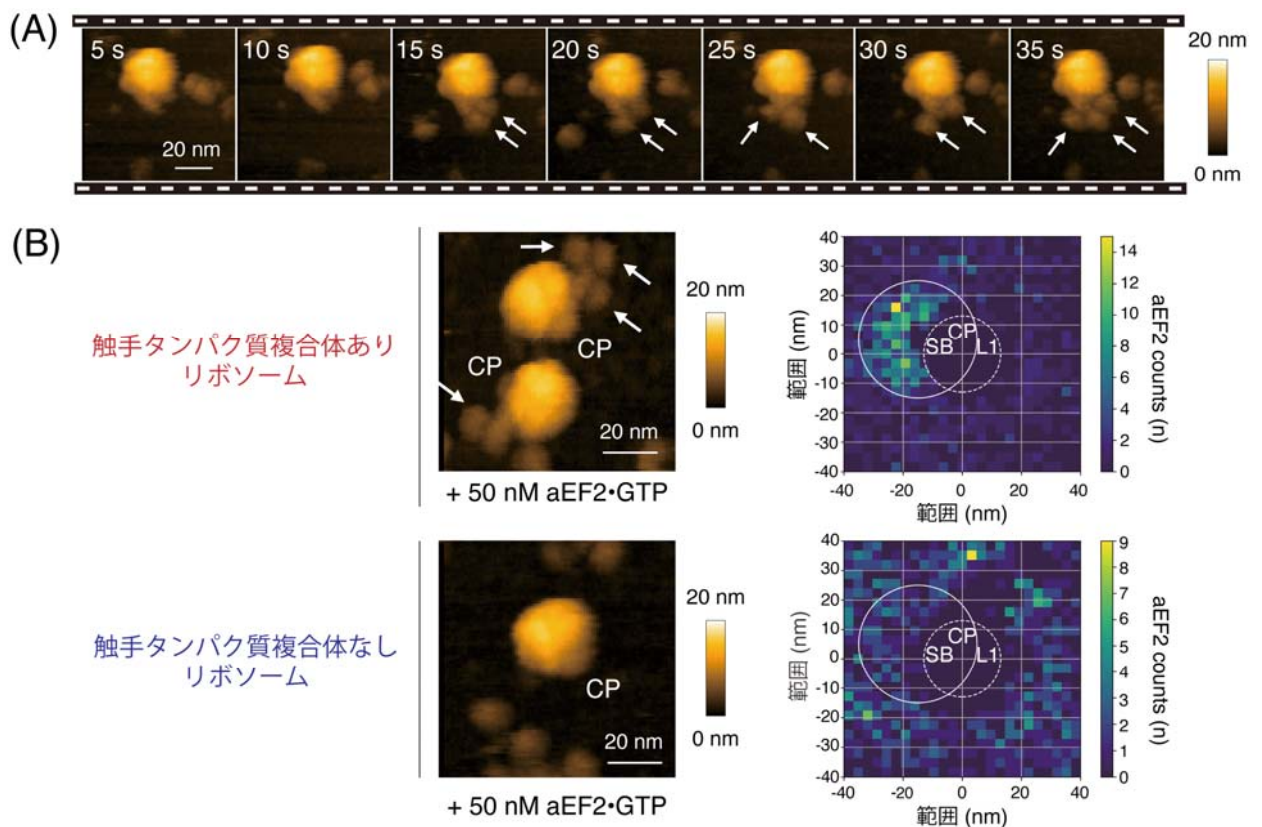
図 2. 触手タンパク質複合体と翻訳因子の相互作用動態
